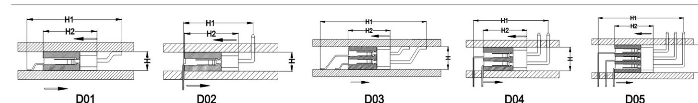
TYPE D(D类)
