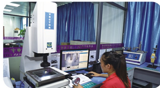
二次元 Binary
