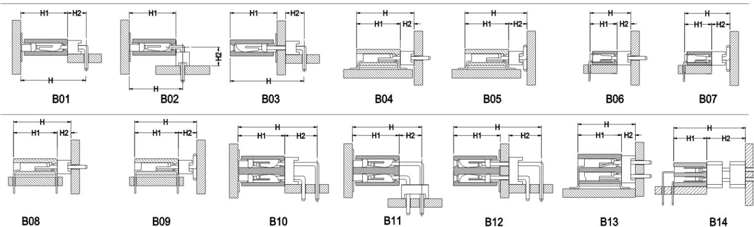
TYPE B(B类)
